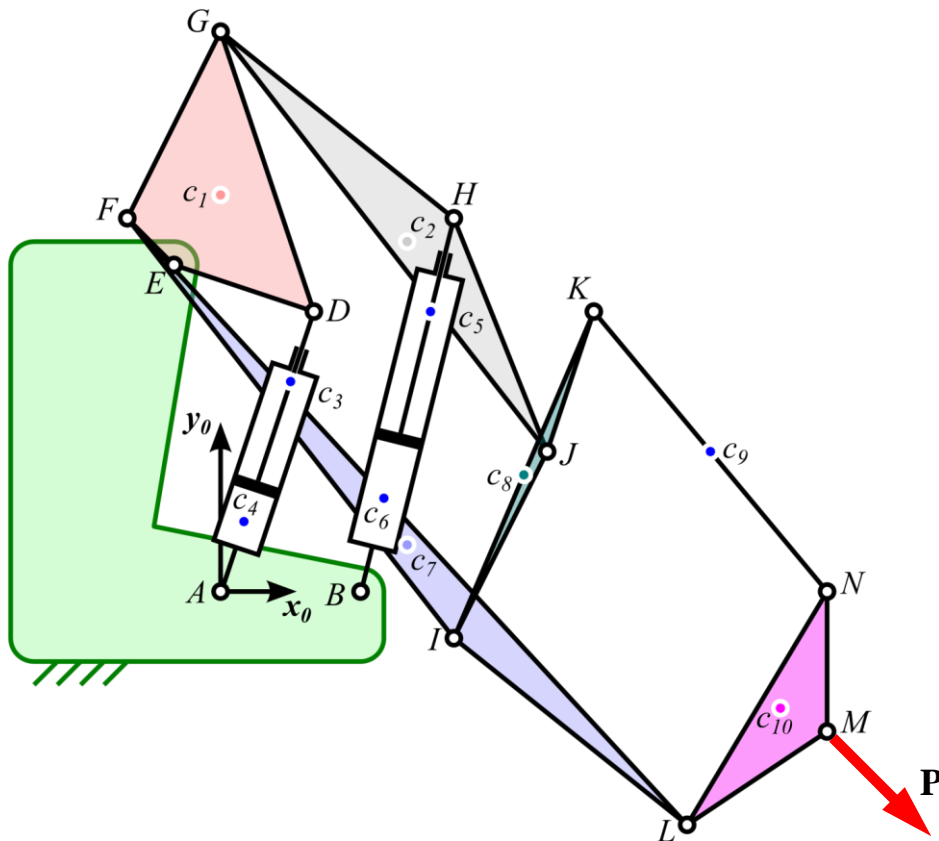
Rysunek 1. Schemat kinematyczny mechanizmu
